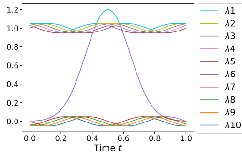
(a) Reordered eigenvalues \lambda_i(t) .
