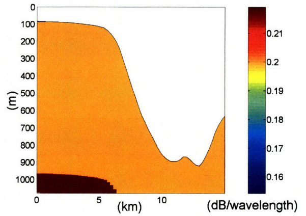
(d) Attenuation coefficient profile of seabed
